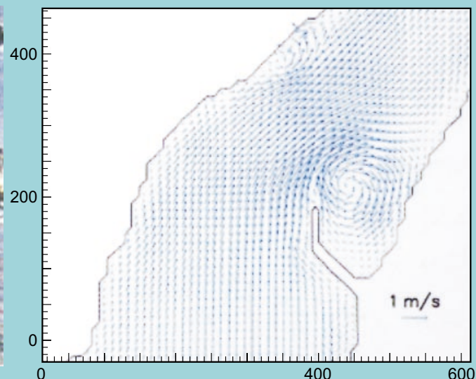
1995 Tsunami Chileno. Izquierda: Una observación de los efectos del tsunami detrás del rompeolas en la bahía Tahauku en las islas Marquesas, Polinesia Francesa, varios miles de kilómetros desde el origen del tsunami. Derecha: Corrientes en la bahía de Tahauku basados en modelación numérica del tsunami chileno. El modelo reproduce las mismas clases de corrientes oceánicas que se ven en la foto.
