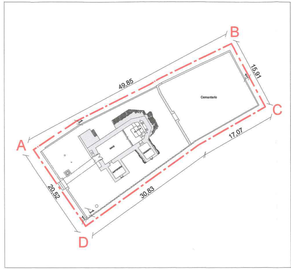
PLANO DE LÍMITES ESCALA GRÁFICA 0 5 10 15 20 m
